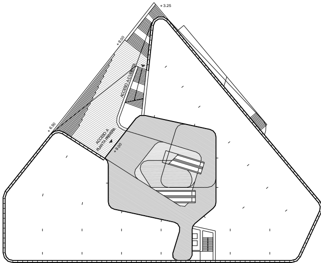
PLANTA PRIMERA. NIVEL + 9.00
