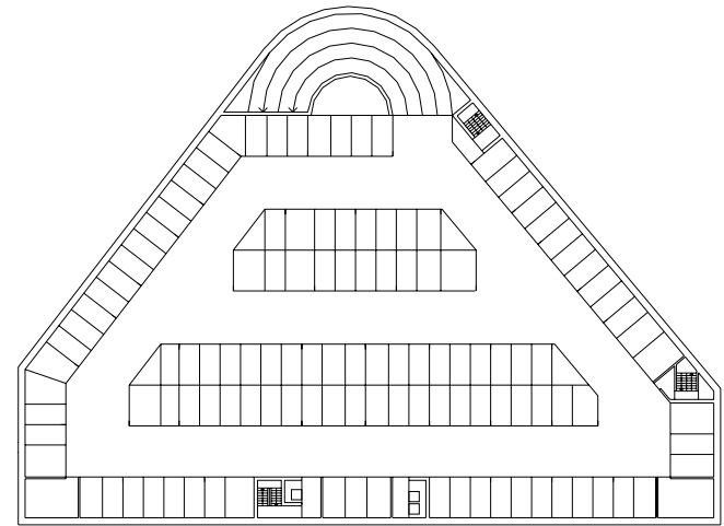
PLANTA SOTANO -4. NIVEL -14.00
