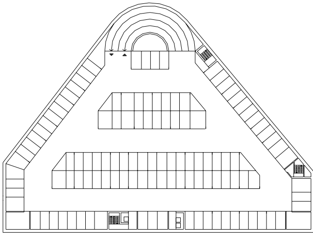
PLANTA SOTANO -3. NIVEL -11.00
