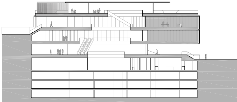
SECCIÓN POR CORE
