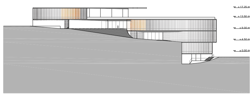
ALZADO MUZATEGI KALEA
