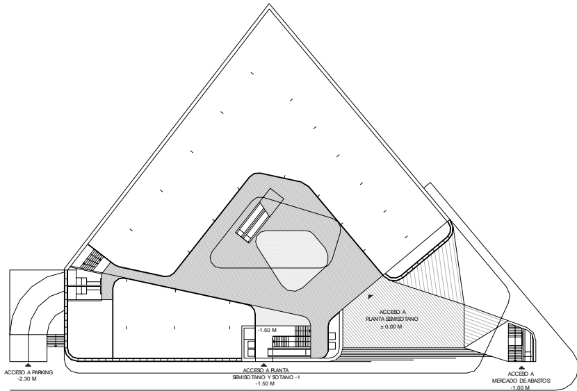
PLANTA SEMISÓTANO. NIVEL ± 0.00
