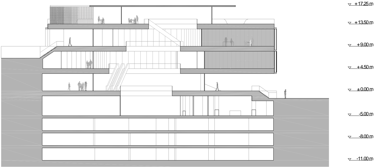
SECCIÓN POR CORE
