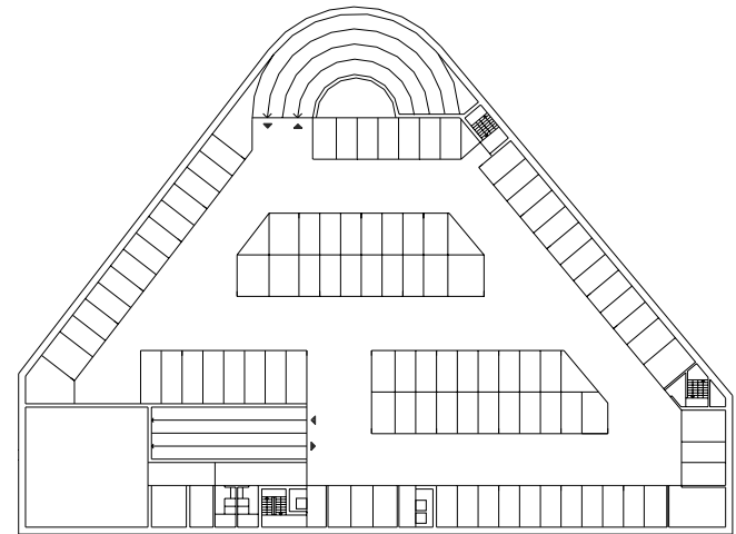
PLANTA SOTANO -2. NIVEL -8.00
